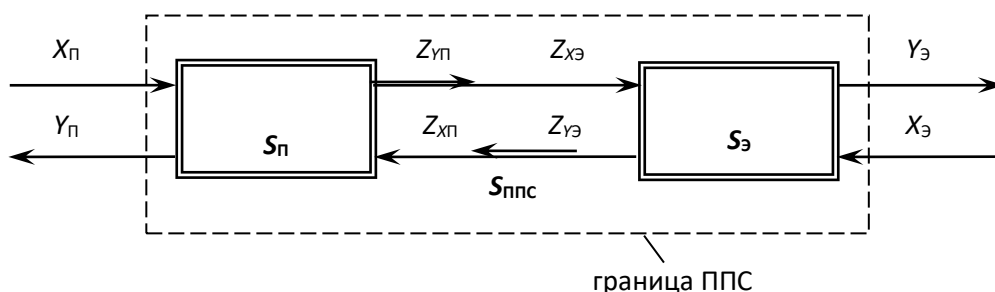
Рис. 1. Структурная схема природно-промышленной системы
